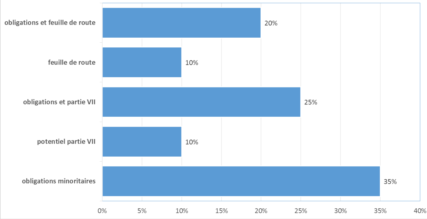
Indicateur composite pour la présence des bureaux fédéraux - poids des composantes
