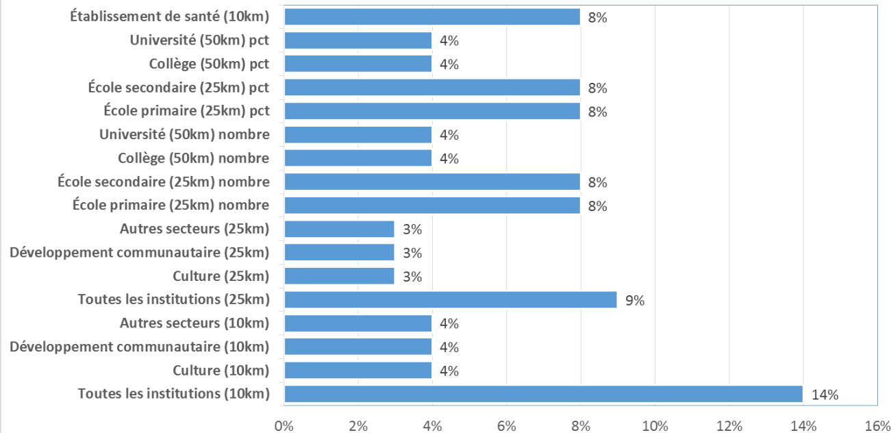
Indicateur composite de proximité institutionnelle - poids des composantes
